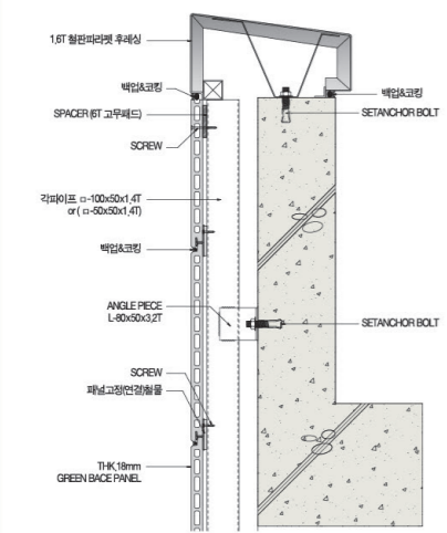
파라펫부위 상세도
