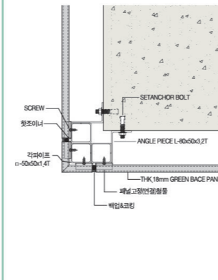
콘크리트구조 - 코너부위 상세도
