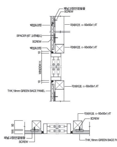
창호 조인트 상세도
